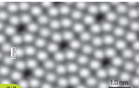
Siliziumoberfläche
